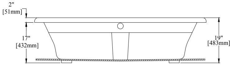
ELEVATION
