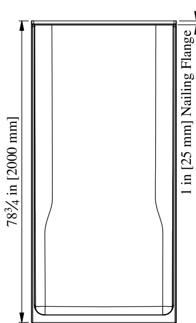
ELEVATION
